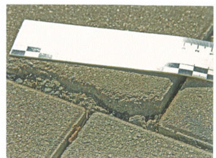
Abb. 8: Kantenschäden an einem Höhenversatz zwischen benachbarten Pflastersteinen
