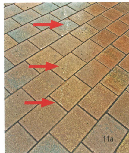
Abb. 11a+b: Nicht sachgerechte Nutzung einer Flächenbefestigung in der Bauzeit
