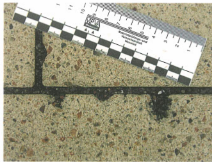
Abb. 1 a+b: Kantenschäden an Betonpflastersteinen
