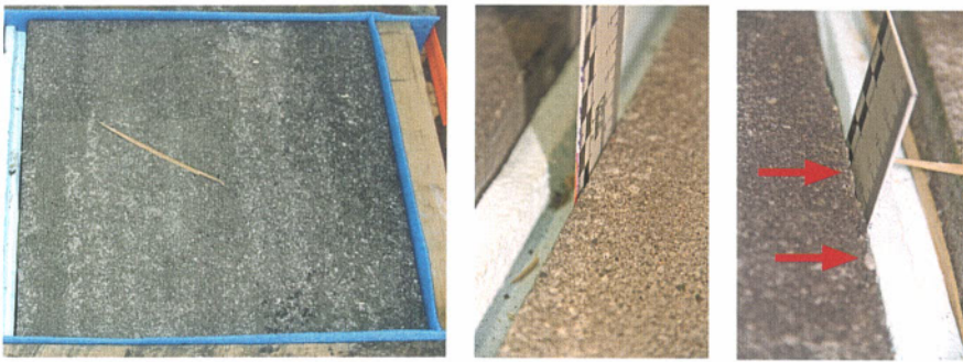
Abb. 13 a+b+c: feine Kantenausbrüche an extrem scharfkantigen Betonplatten
